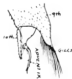
Fig. 223. Tip of abdomen.
